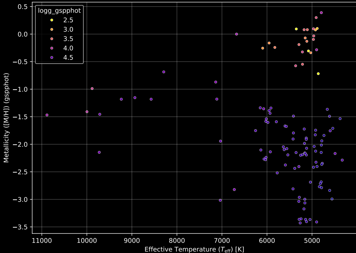
Gaia Cluster: [Czernik_26] Stellar Population Parameters (n= 117)
