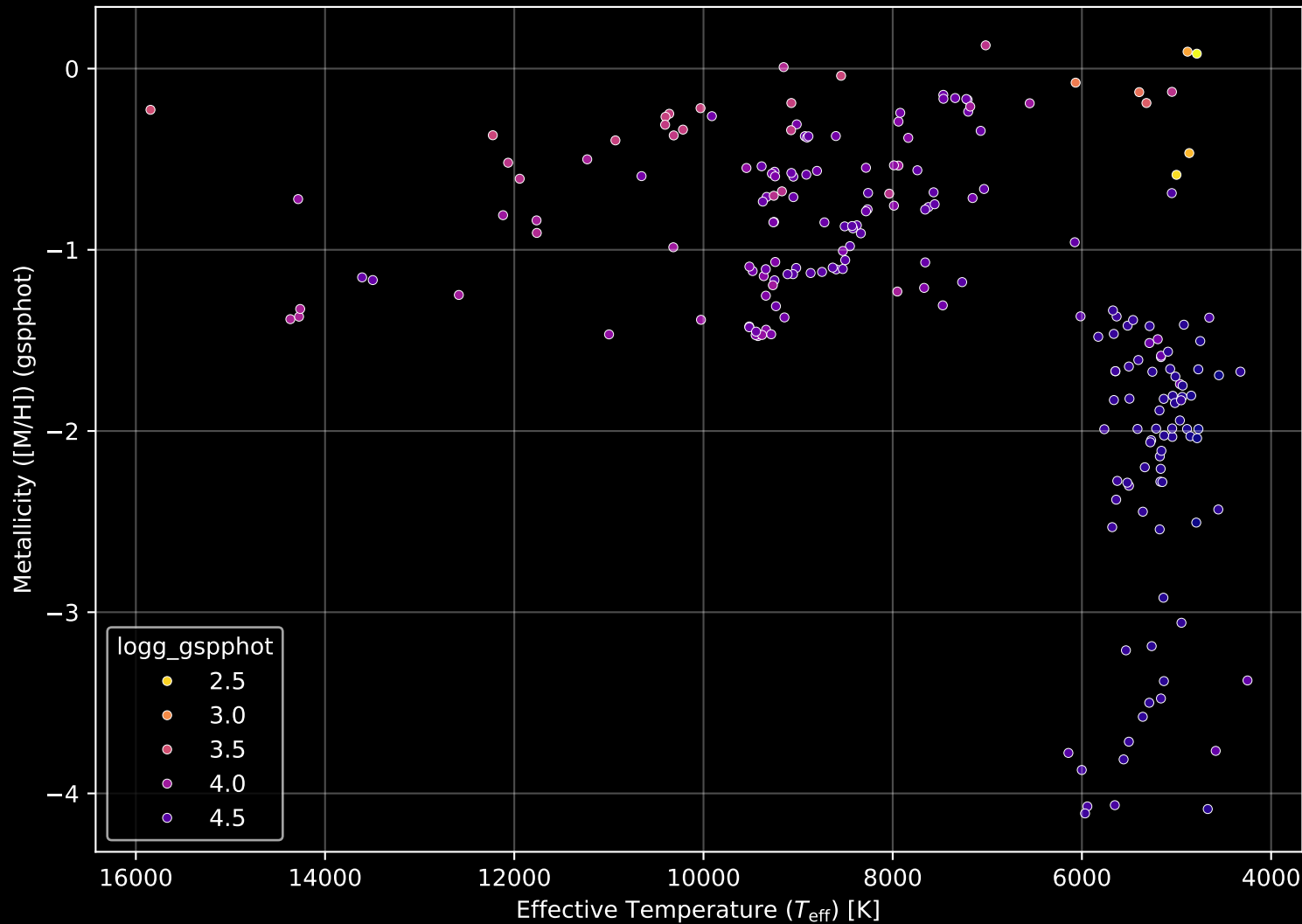
Gaia Cluster: [Czernik_31] Stellar Population Parameters (n= 215)
