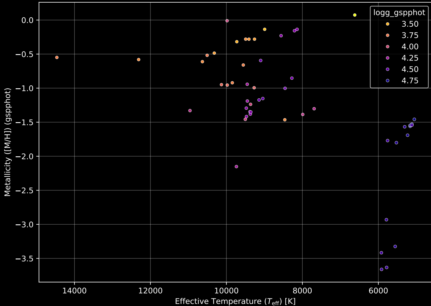
Gaia Cluster: [Czernik_8] Stellar Population Parameters (n= 54)
