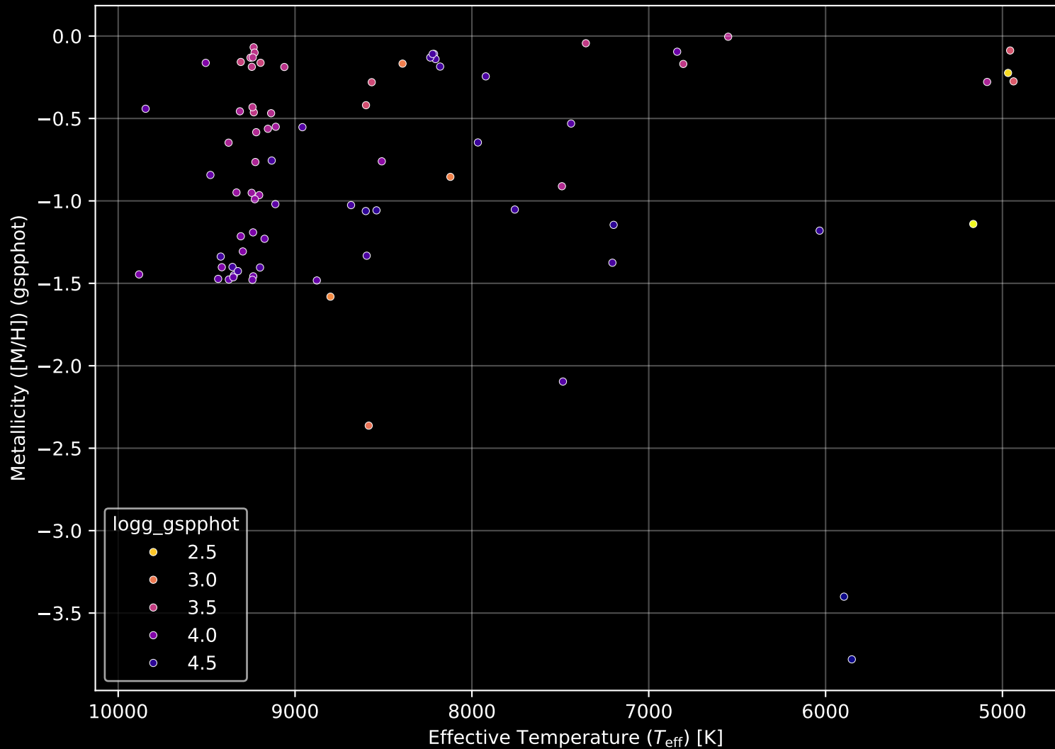
Gaia Cluster: [Czernik_9] Stellar Population Parameters (n= 80)
