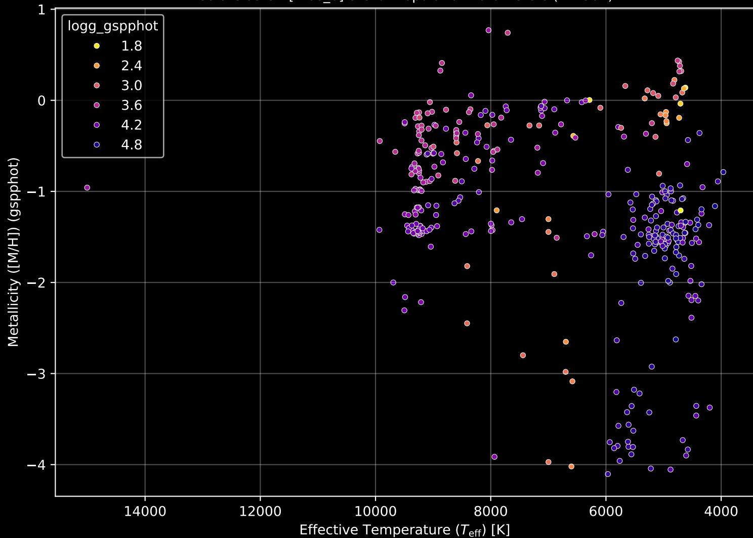
Gaia Cluster: [Dias_6] Stellar Population Parameters (n= 384)
