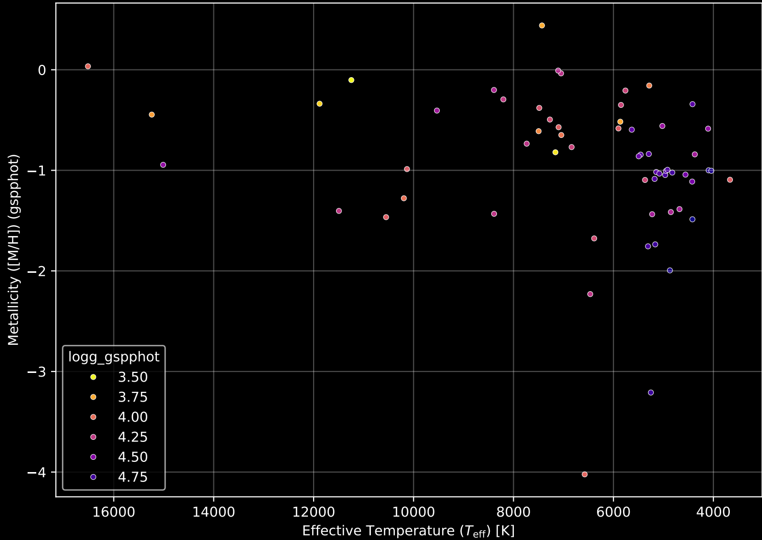
Gaia Cluster: [Dolidze_16] Stellar Population Parameters (n= 61)
