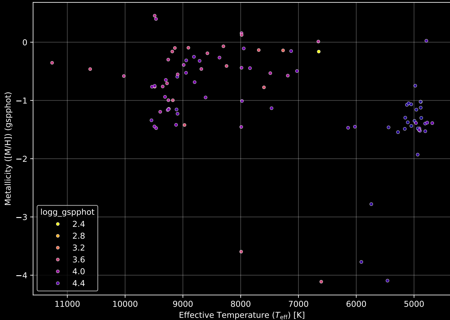
Gaia Cluster: [Dolidze_5] Stellar Population Parameters (n= 95)
