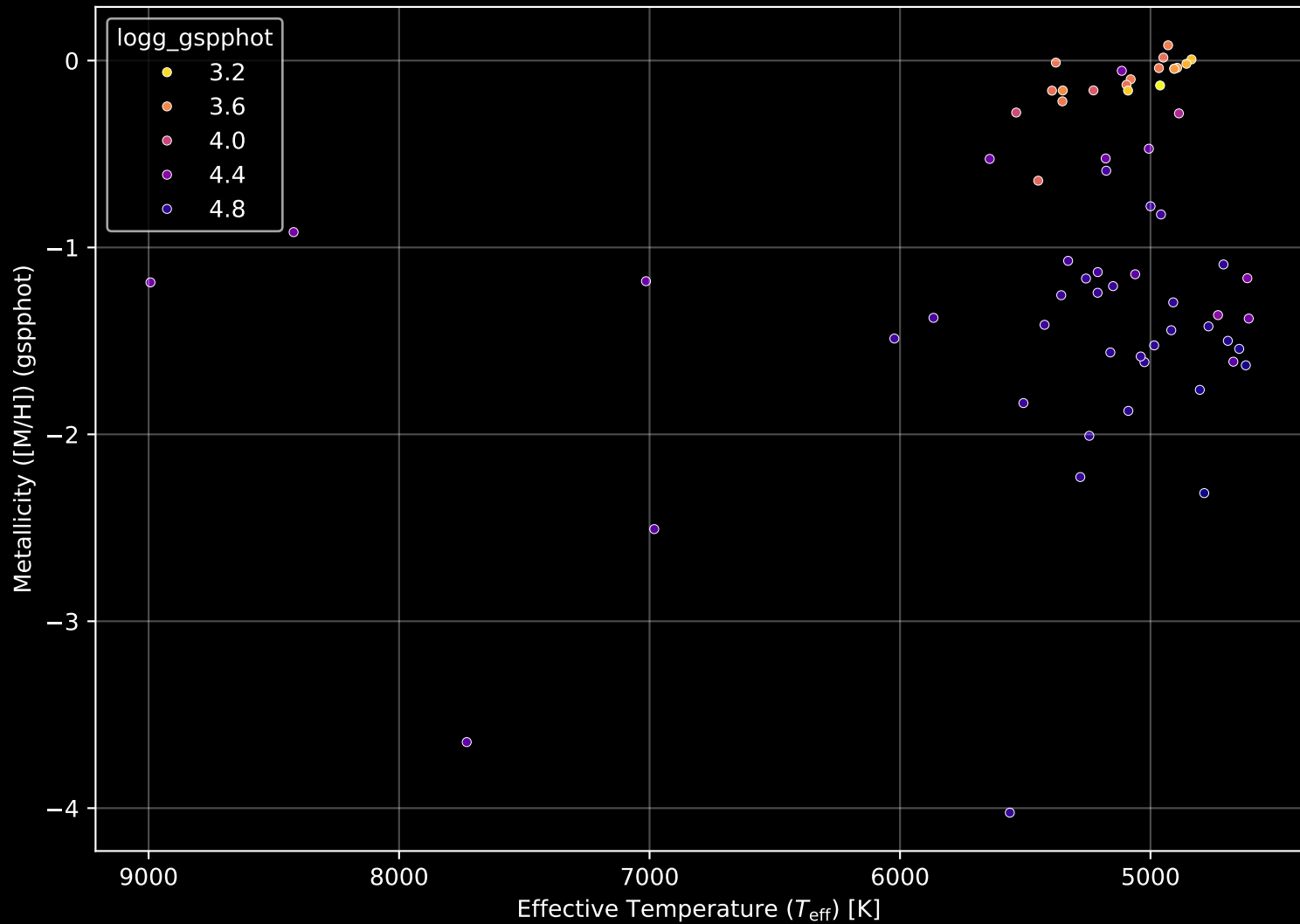
Gaia Cluster: [ESO_092_05] Stellar Population Parameters (n= 64)
