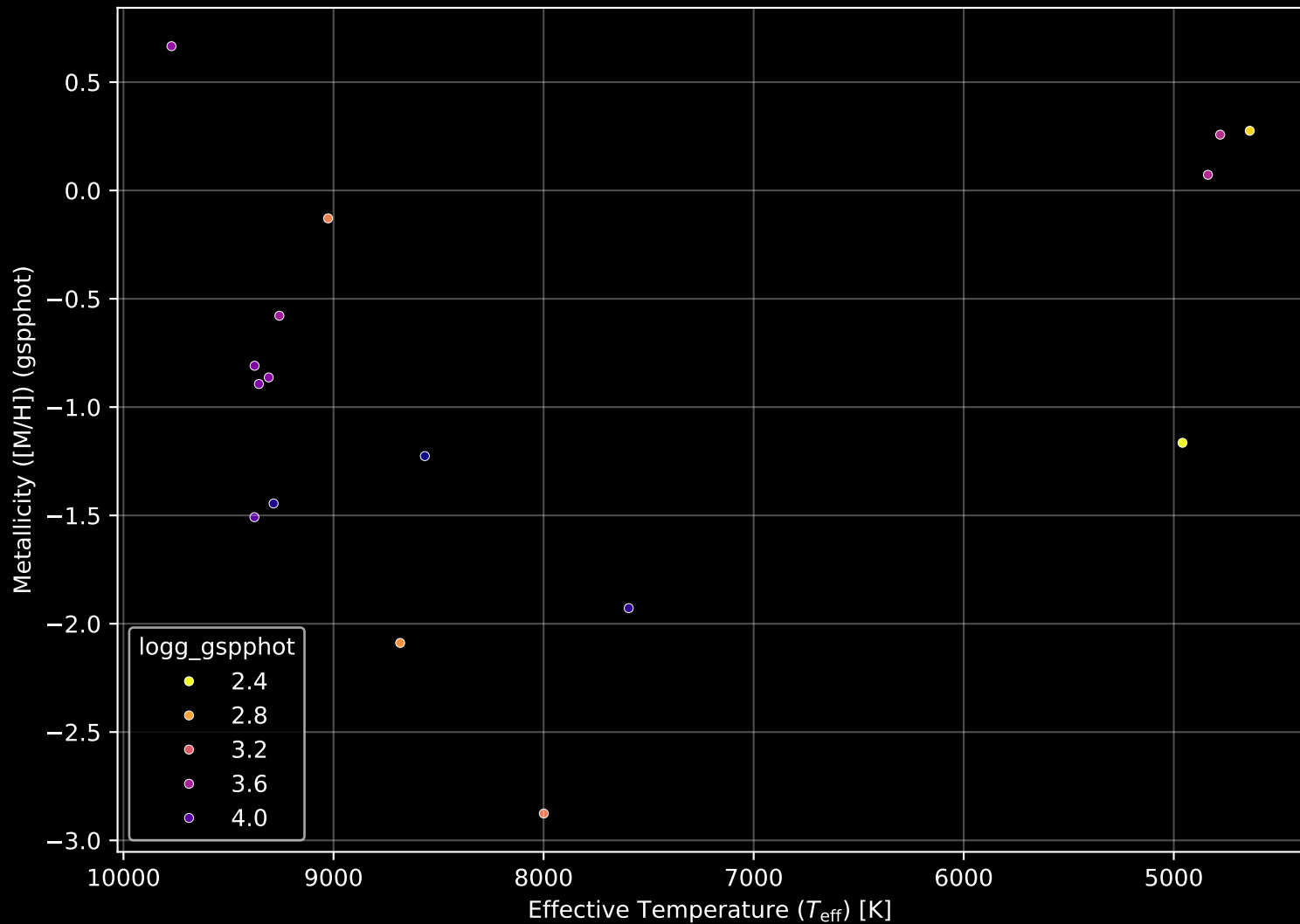
Gaia Cluster: [ESO_211_09] Stellar Population Parameters (n= 16)
