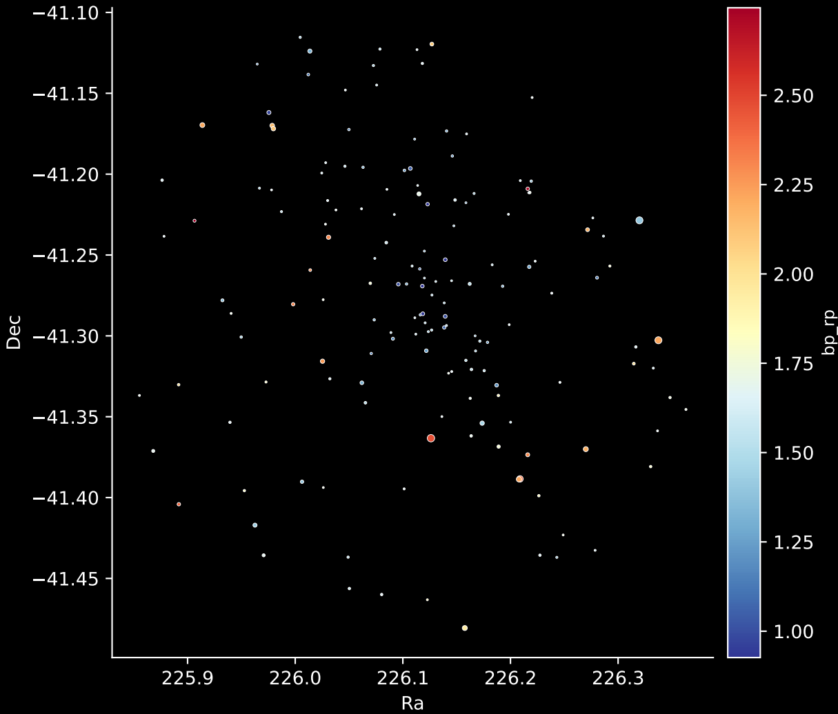
Gaia Cluster: [ESO_312_03] Stars: 159
