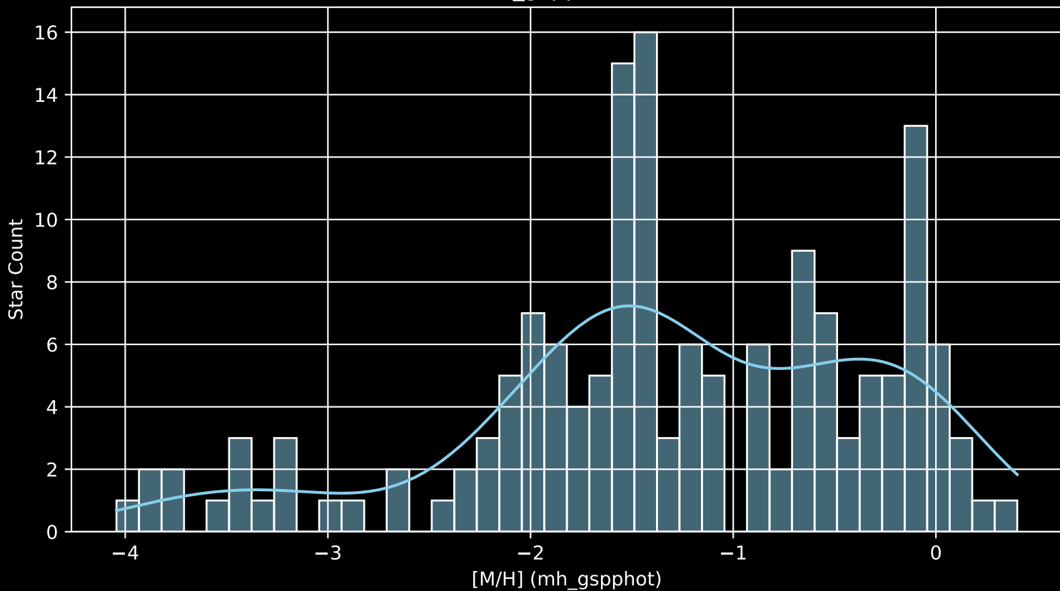
Gaia Cluster: [ESO_312_03 [M/H] (mh_gspphot) (n= 156)
