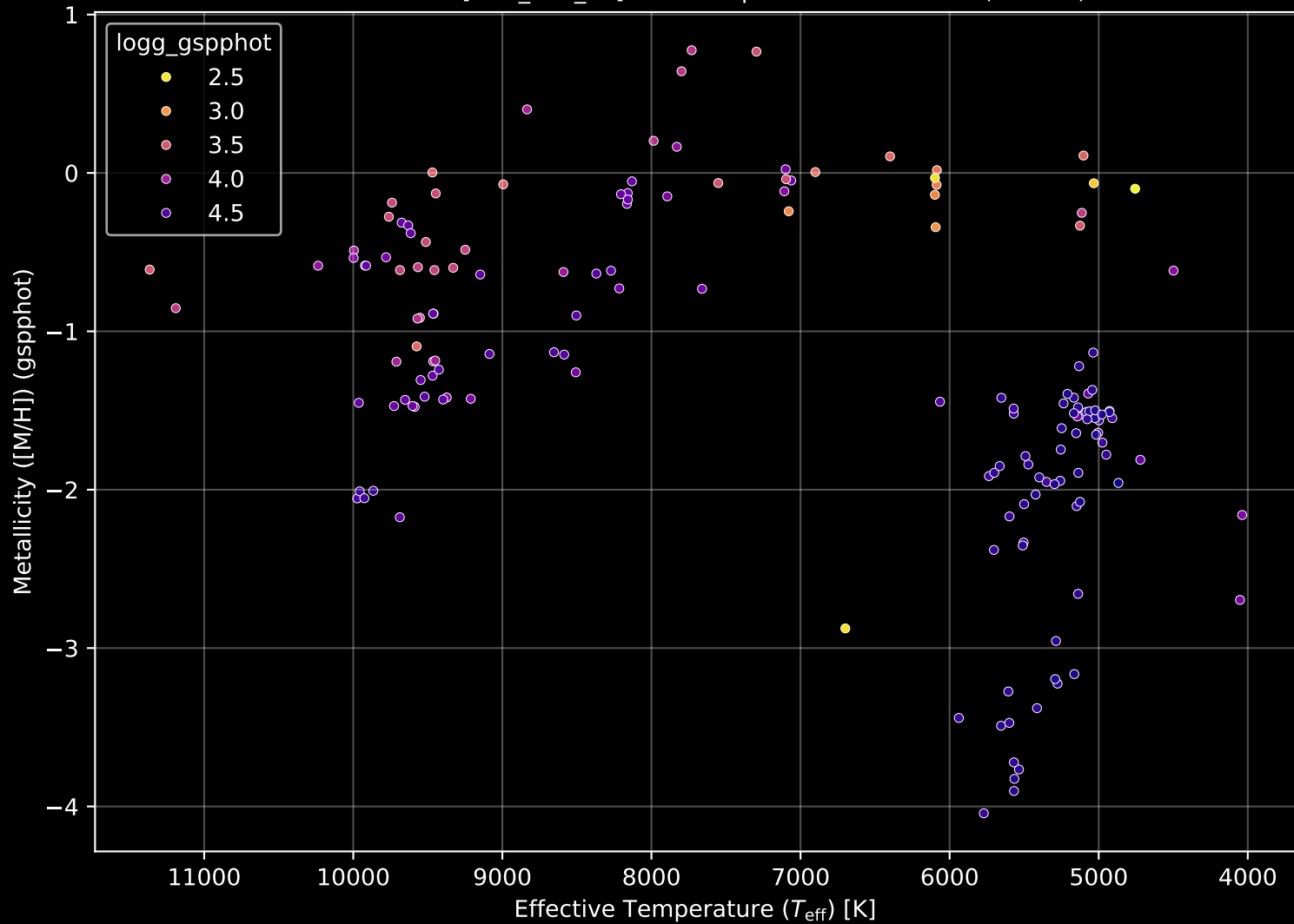
Gaia Cluster: [ESO_312_03] Stellar Population Parameters (n= 159)
