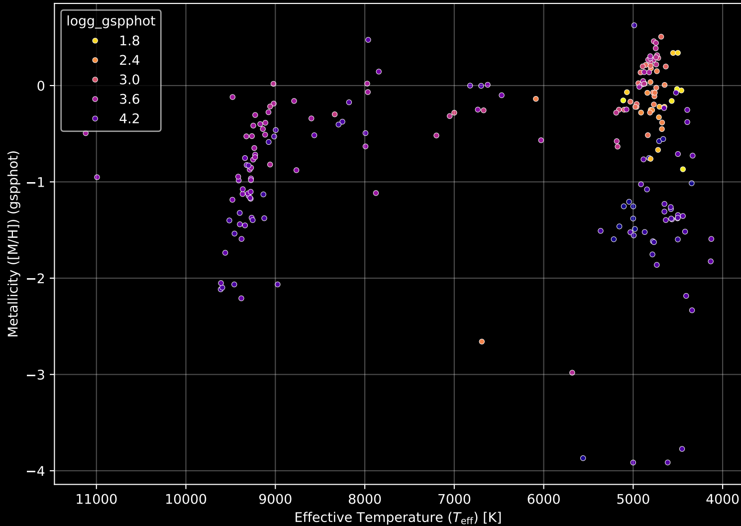
Gaia Cluster: [FSR_0123] Stellar Population Parameters (n= 201)
