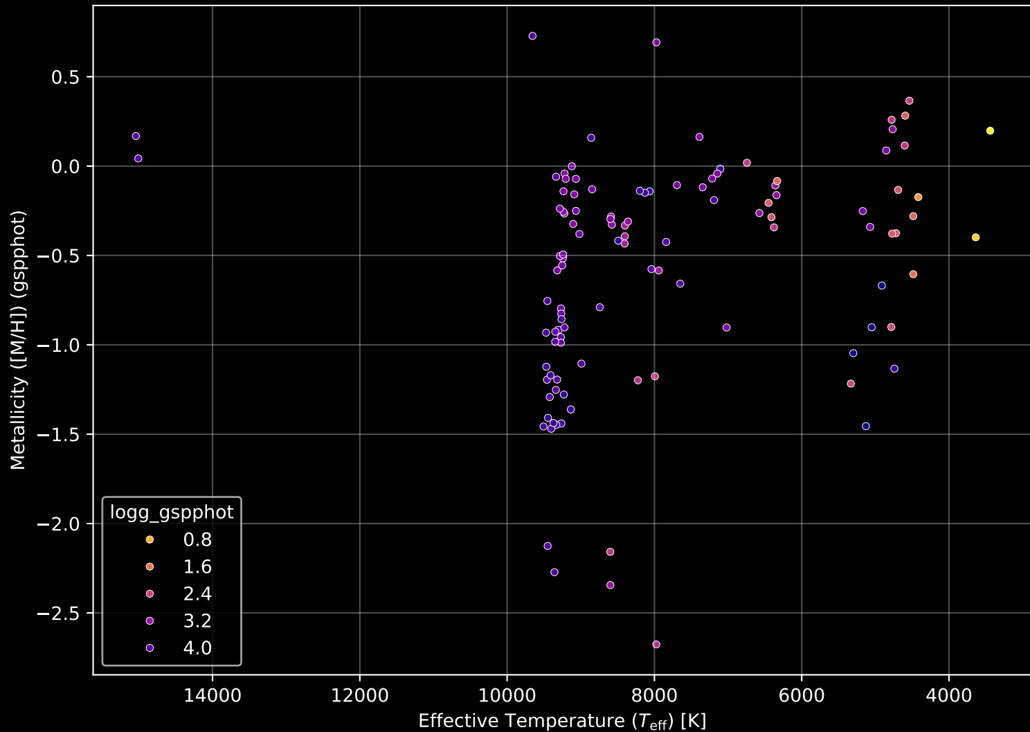
Gaia Cluster: [FSR_0154] Stellar Population Parameters (n= 113)
