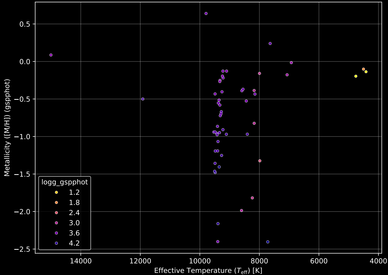
Gaia Cluster: [FSR_0158] Stellar Population Parameters (n= 53)
