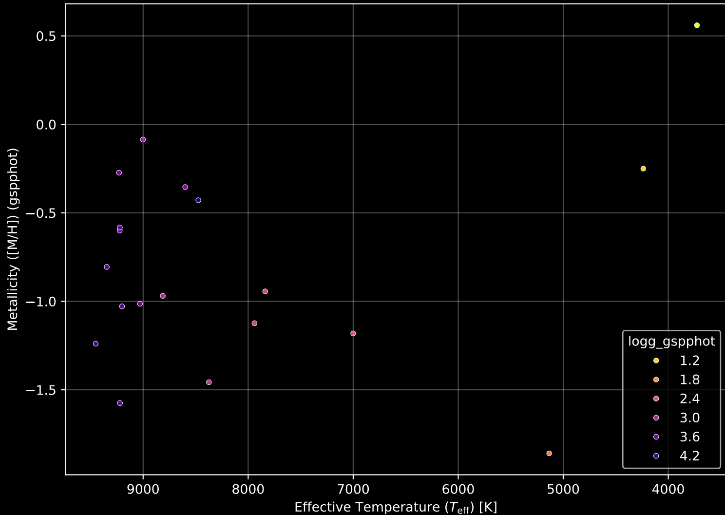
Gaia Cluster: [FSR_0238] Stellar Population Parameters (n= 19)
