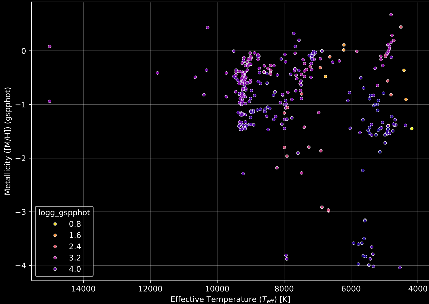
Gaia Cluster: [FSR_0336] Stellar Population Parameters (n= 358)
