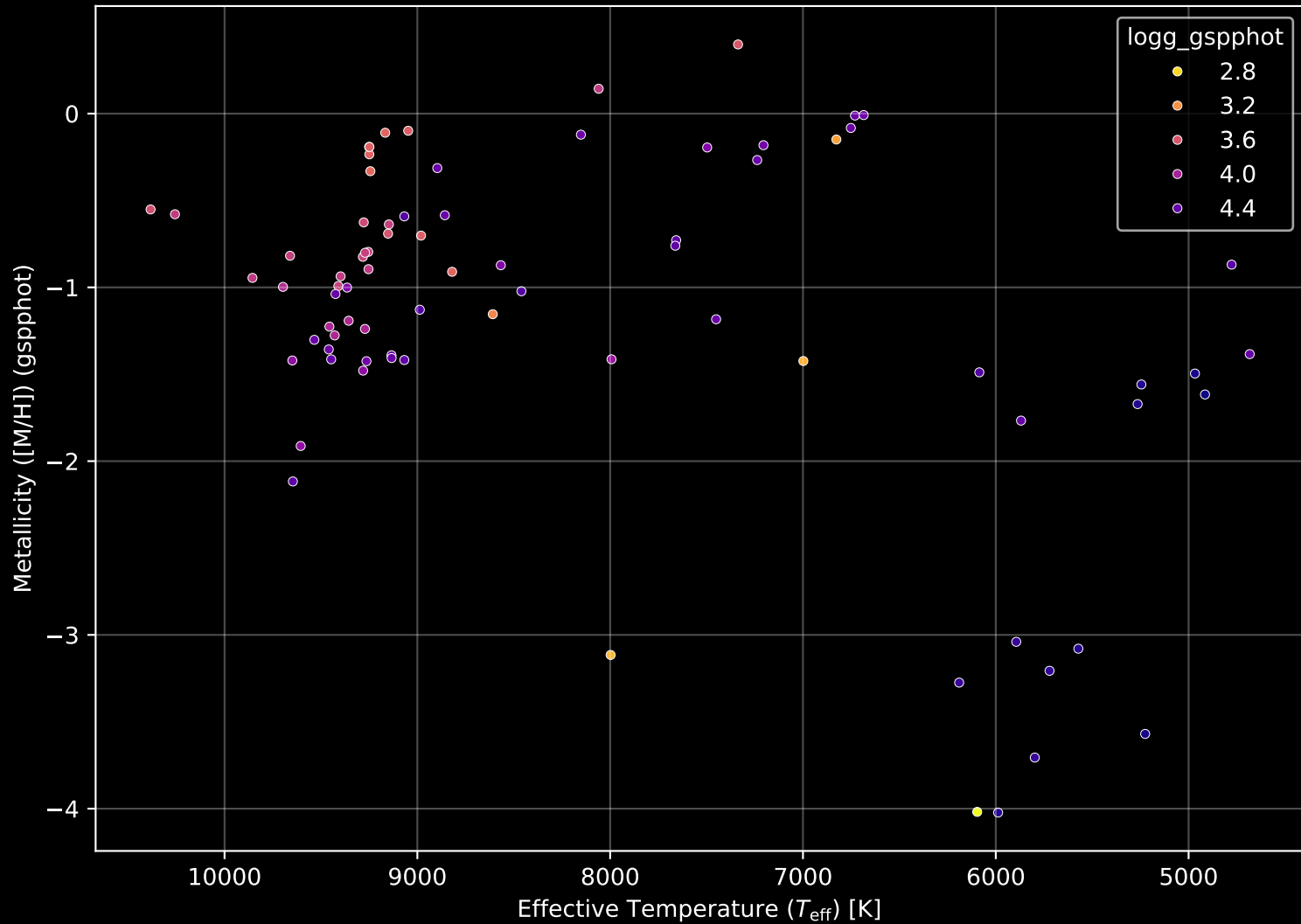
Gaia Cluster: [FSR_0448] Stellar Population Parameters (n= 78)
