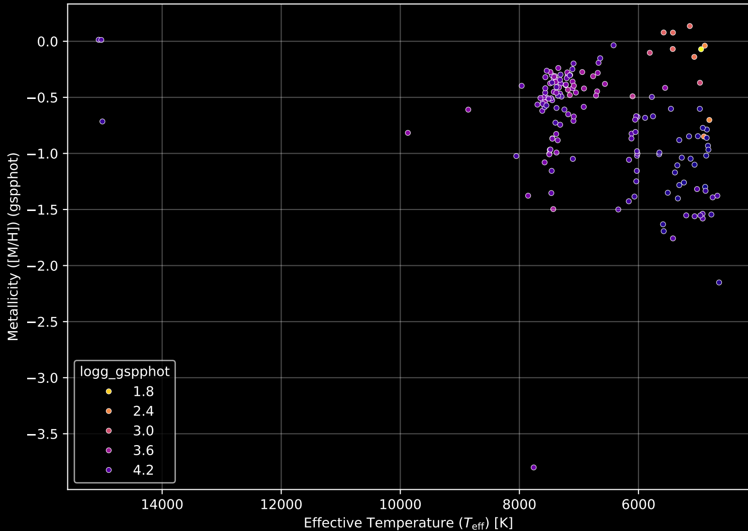
Gaia Cluster: [FSR_0496] Stellar Population Parameters (n= 163)
