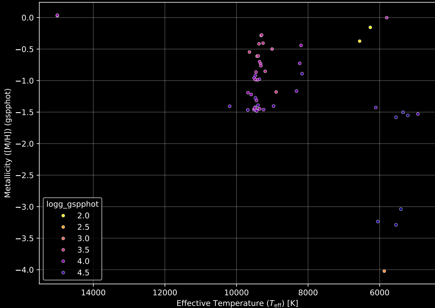
Gaia Cluster: [FSR_0524] Stellar Population Parameters (n= 54)
