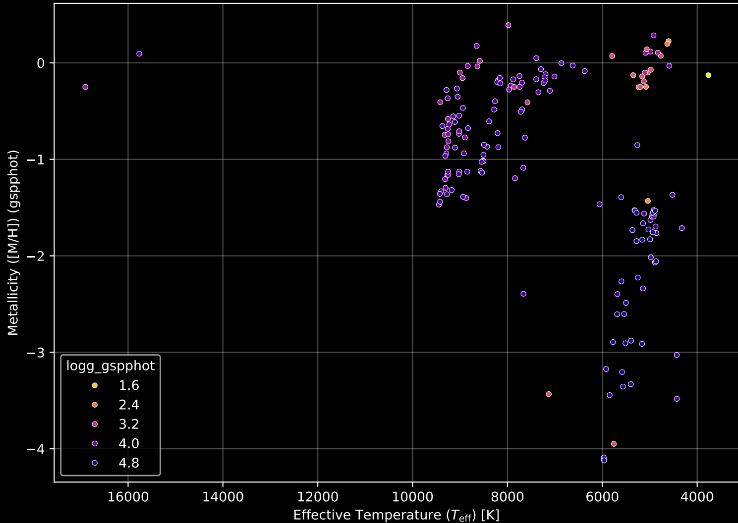
Gaia Cluster: [FSR_0558] Stellar Population Parameters (n= 167)
