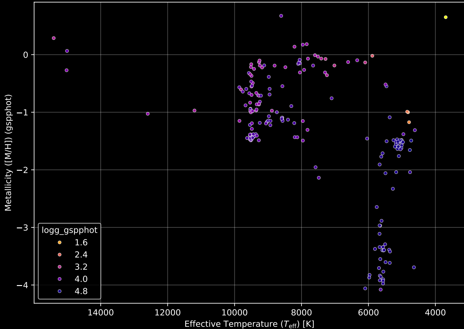
Gaia Cluster: [FSR_0826] Stellar Population Parameters (n= 194)
