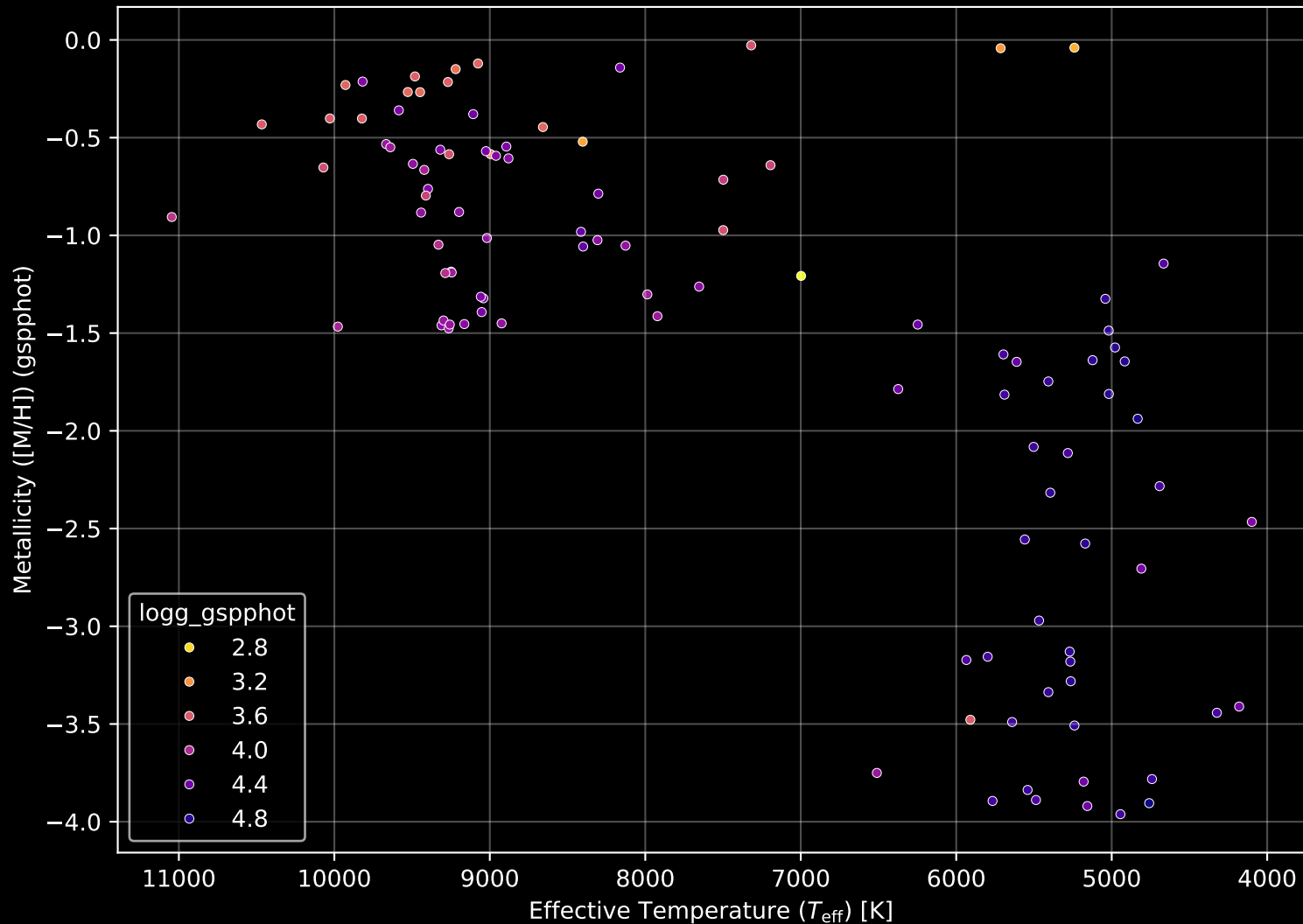
Gaia Cluster: [FSR_0883] Stellar Population Parameters (n= 106)
