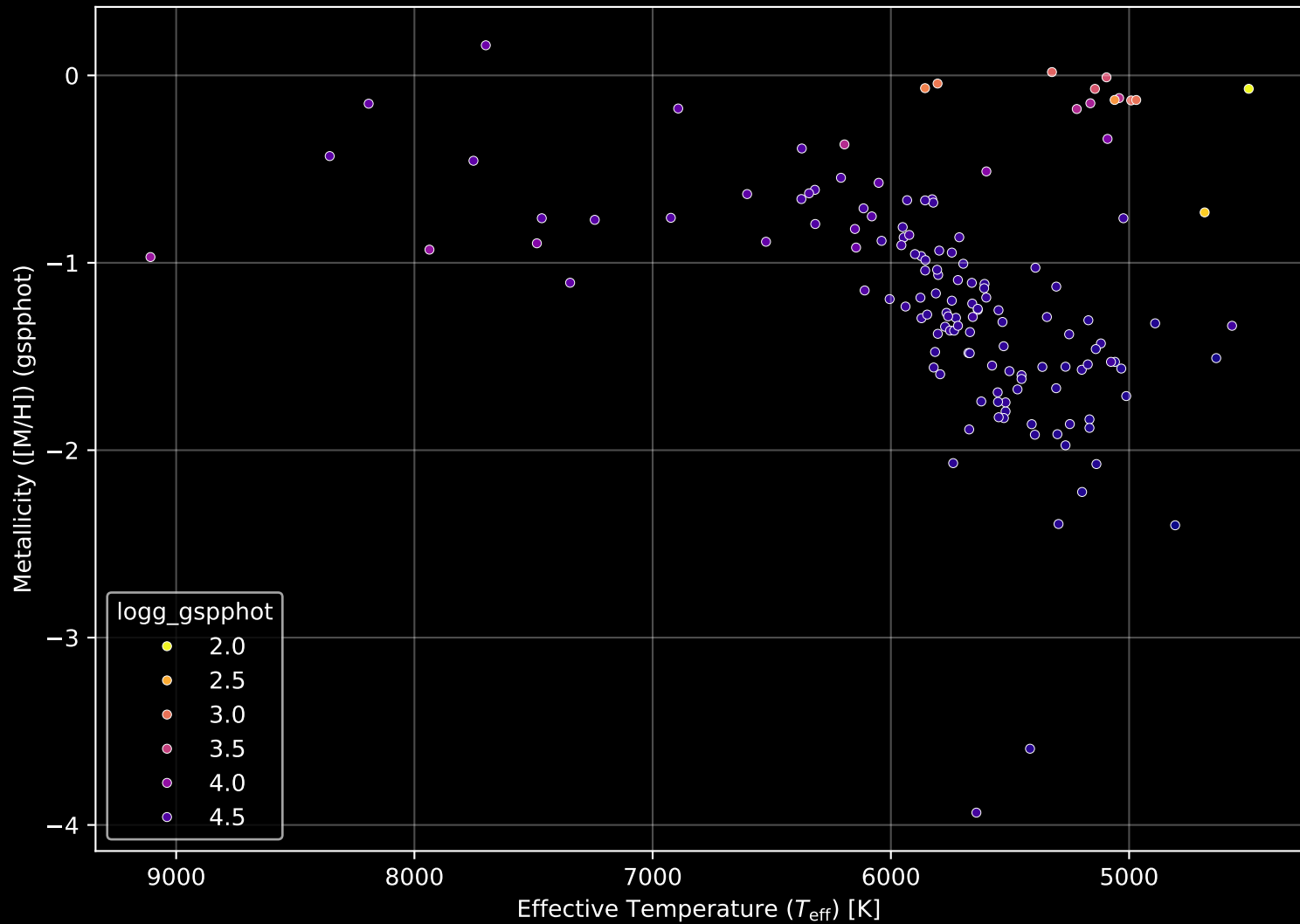
Gaia Cluster: [FSR_1083] Stellar Population Parameters (n= 141)
