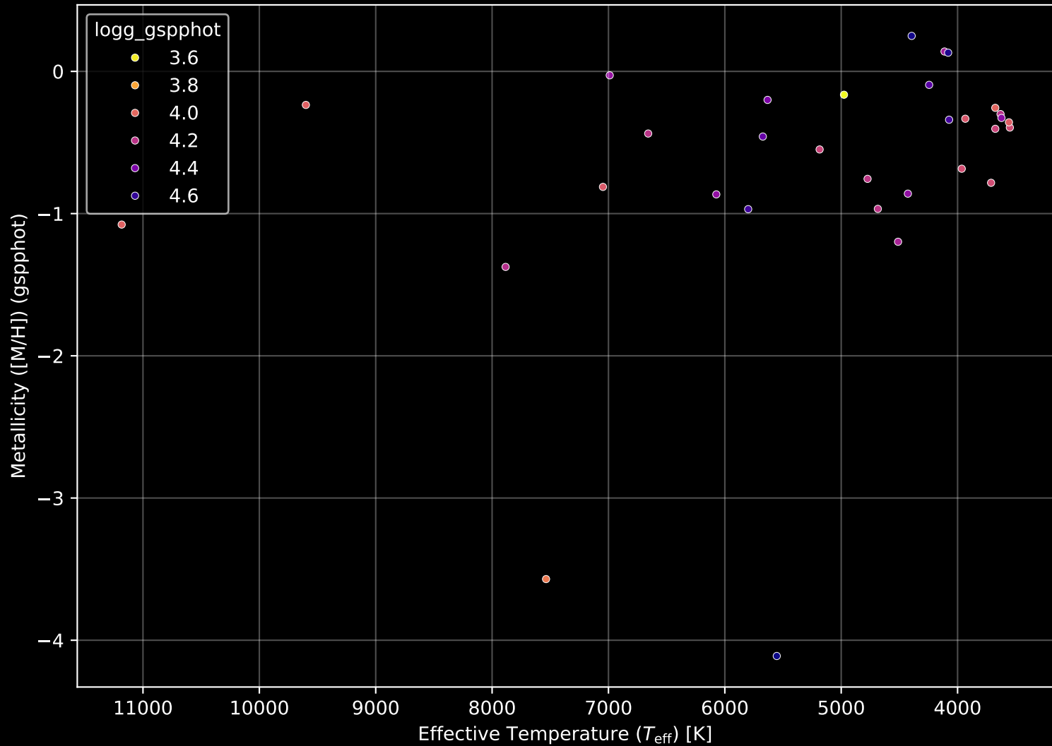
Gaia Cluster: [FSR_1117] Stellar Population Parameters (n= 32)
