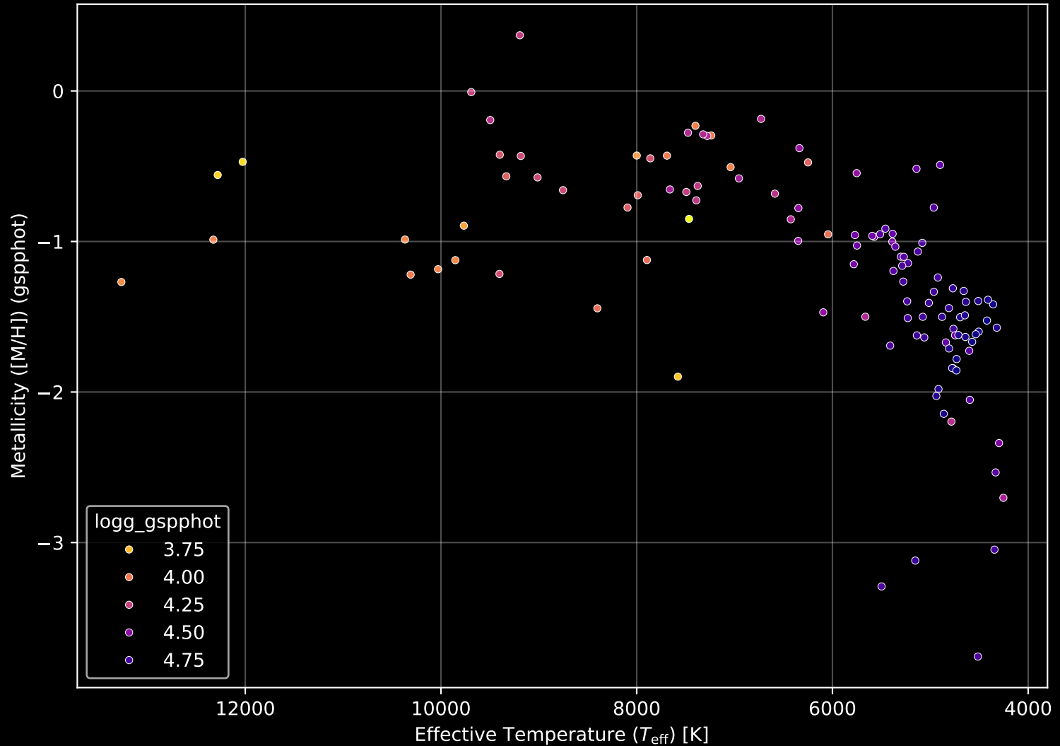
Gaia Cluster: [FSR_1144] Stellar Population Parameters (n= 117)
