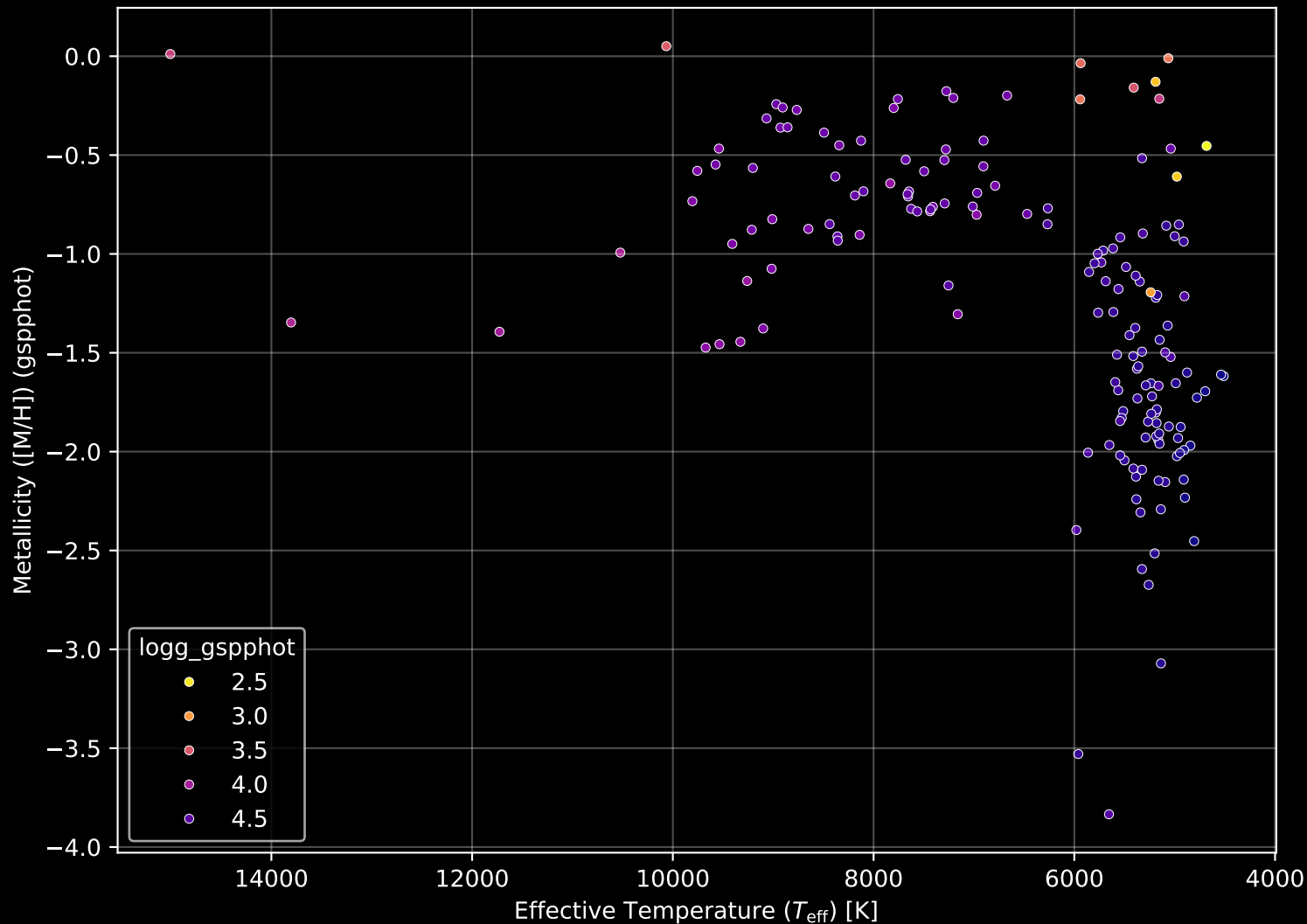
Gaia Cluster: [FSR_1153] Stellar Population Parameters (n= 165)
