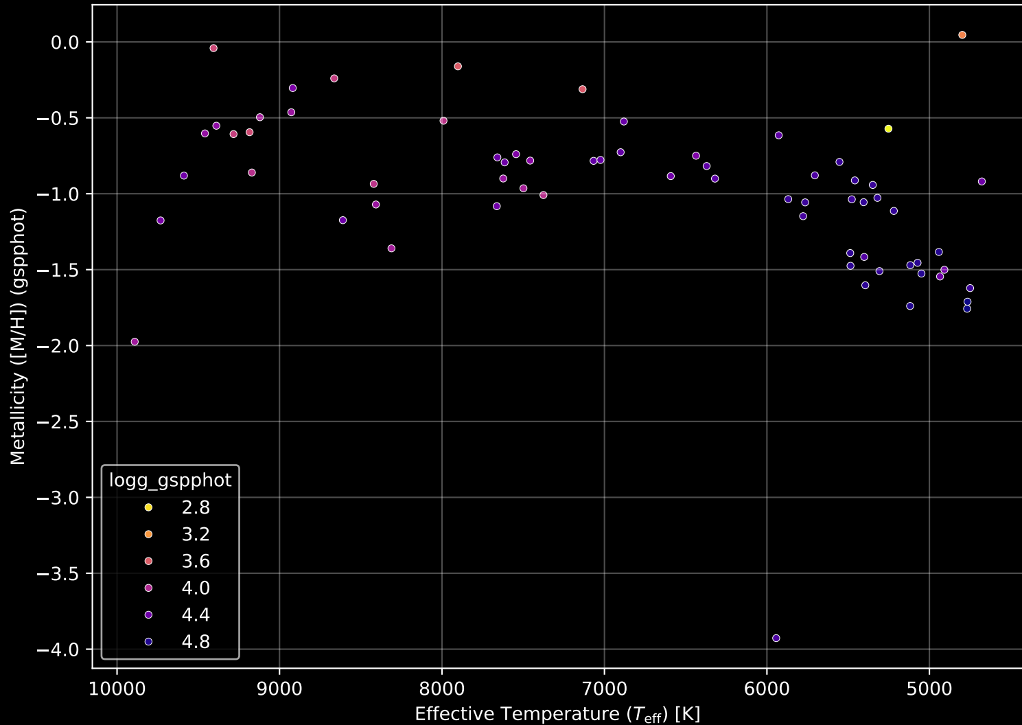
Gaia Cluster: [FSR_1284] Stellar Population Parameters (n= 67)
