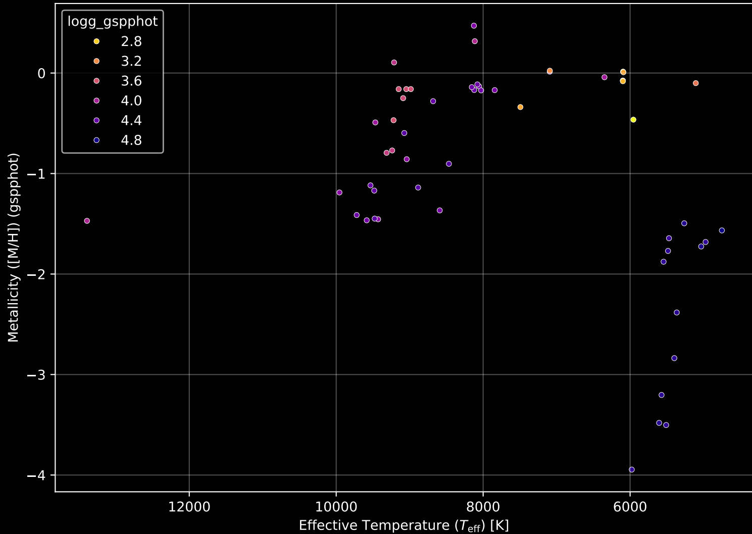
Gaia Cluster: [FSR_1380] Stellar Population Parameters (n= 55)
