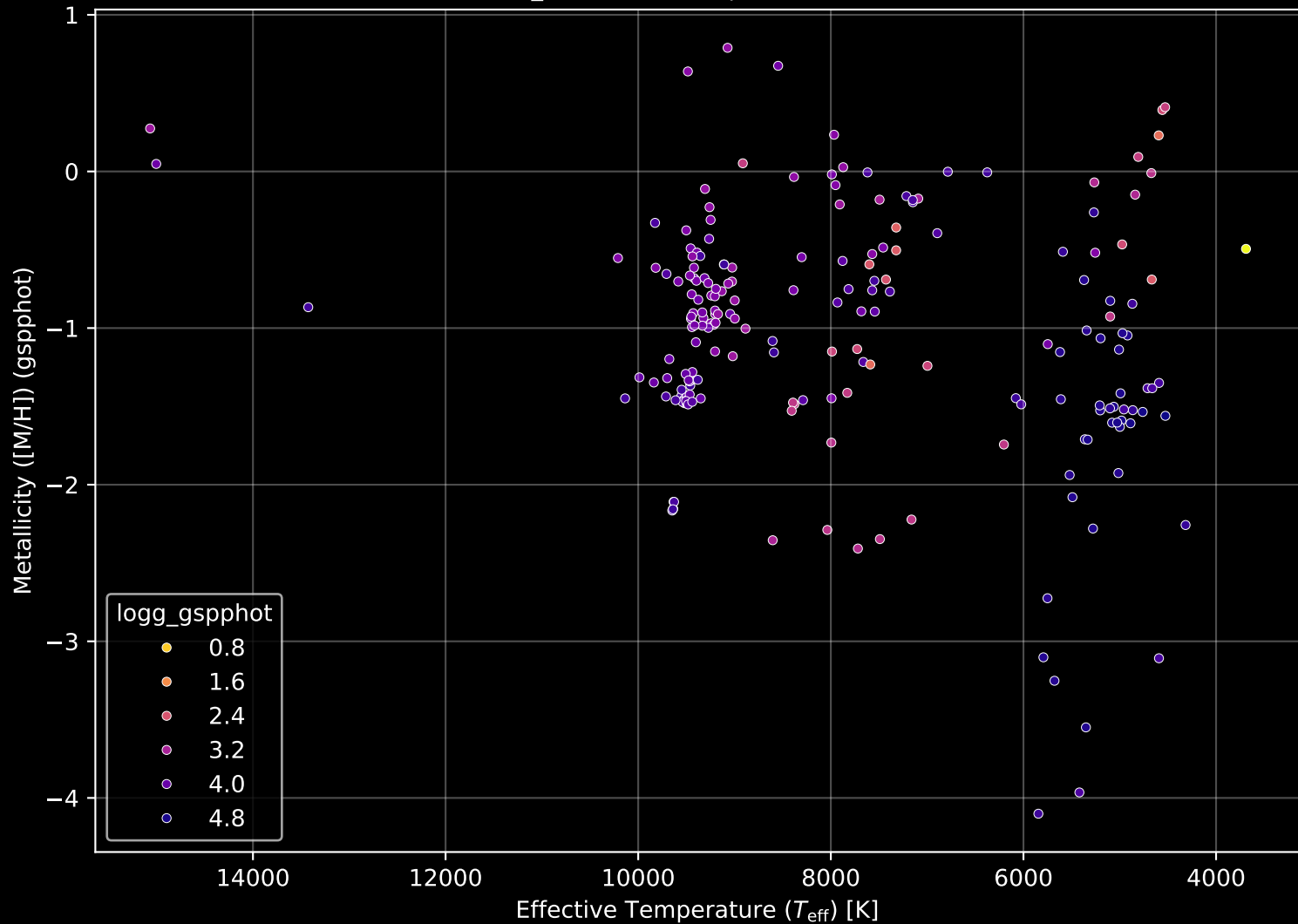
Gaia Cluster: [FSR_1586] Stellar Population Parameters (n= 207)
