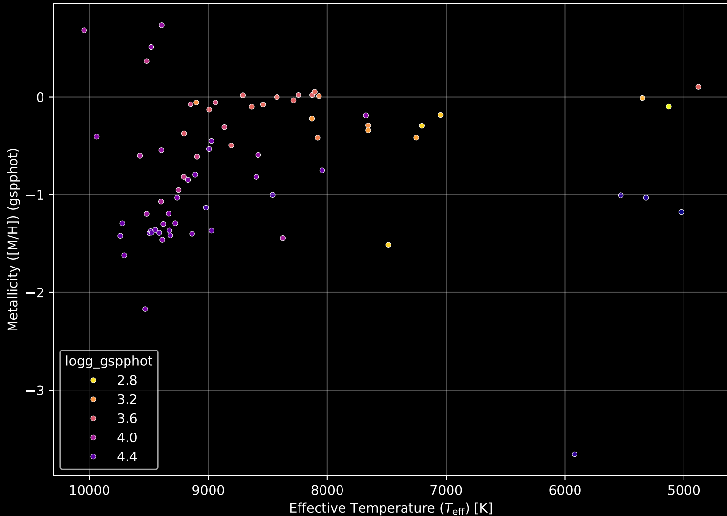
Gaia Cluster: [FSR_1663] Stellar Population Parameters (n= 72)
