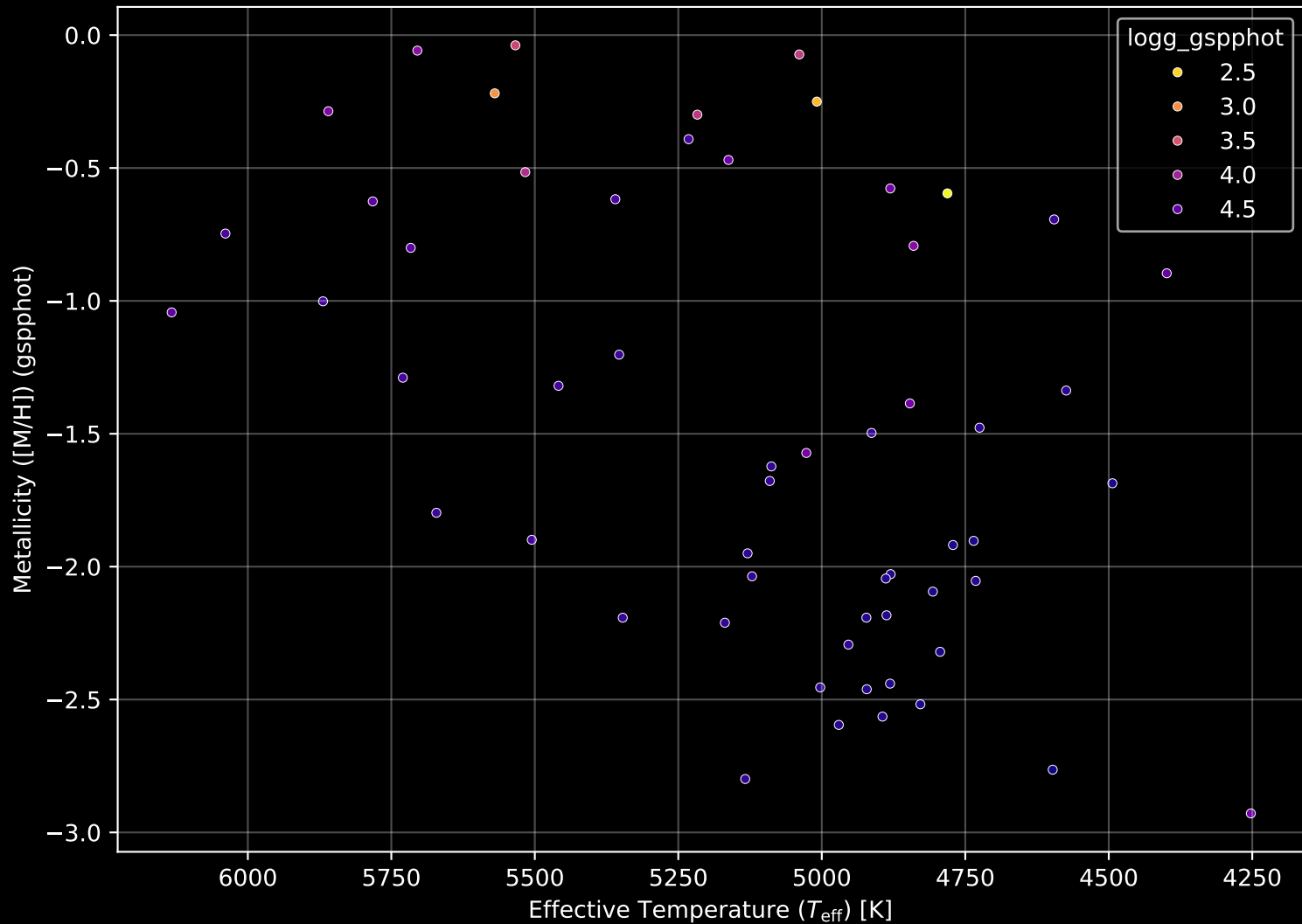
Gaia Cluster: [Gaia_2] Stellar Population Parameters (n= 57)
