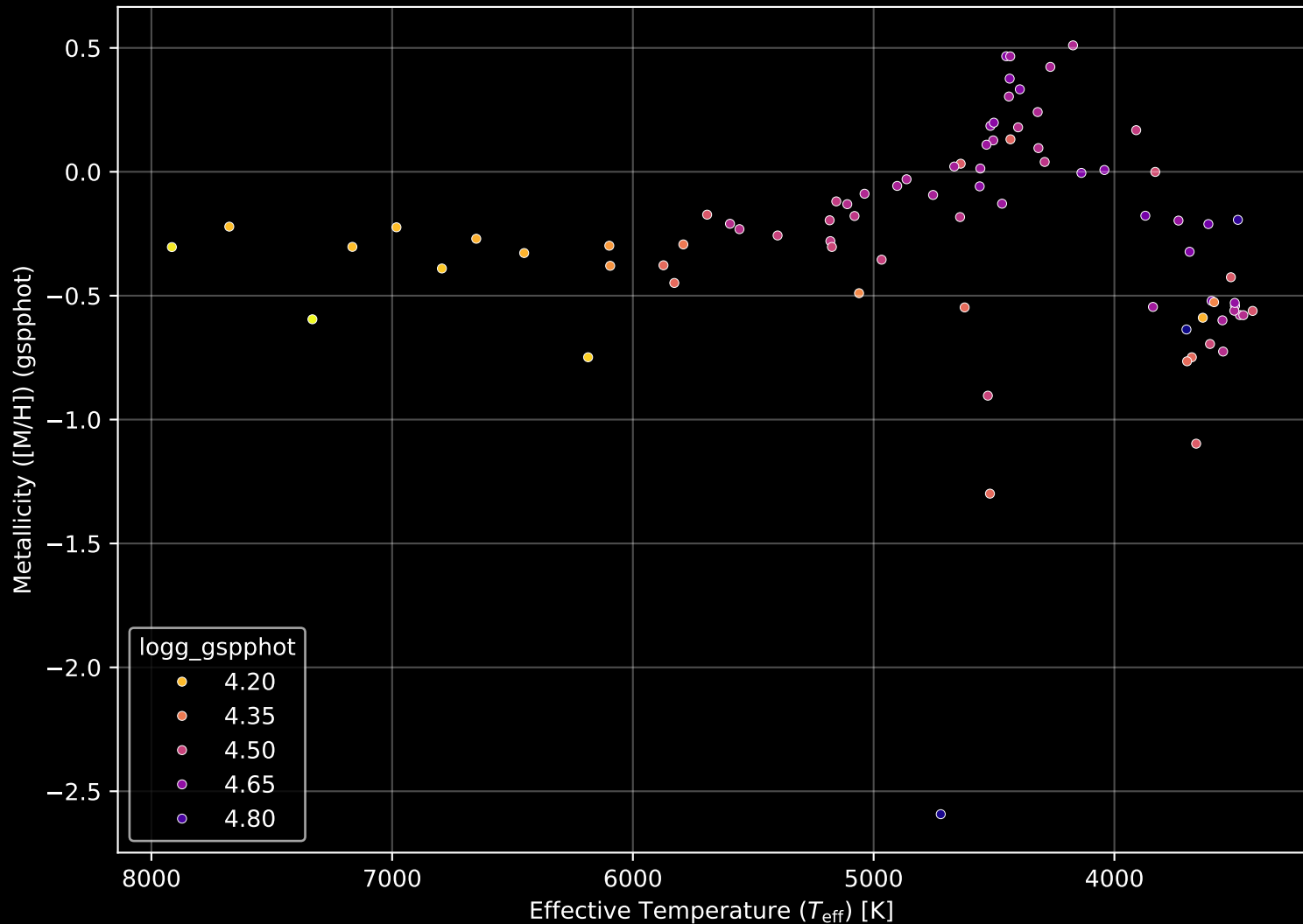
Gaia Cluster: [Gulliver_20] Stellar Population Parameters (n= 83)
