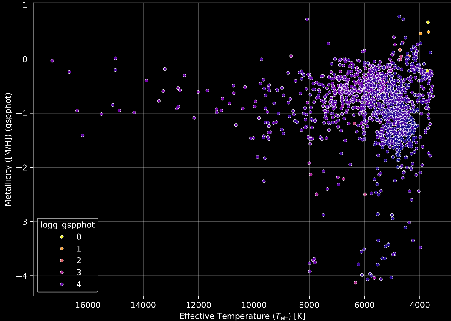
Gaia Cluster: [Gulliver_29] Stellar Population Parameters (n= 1545)
