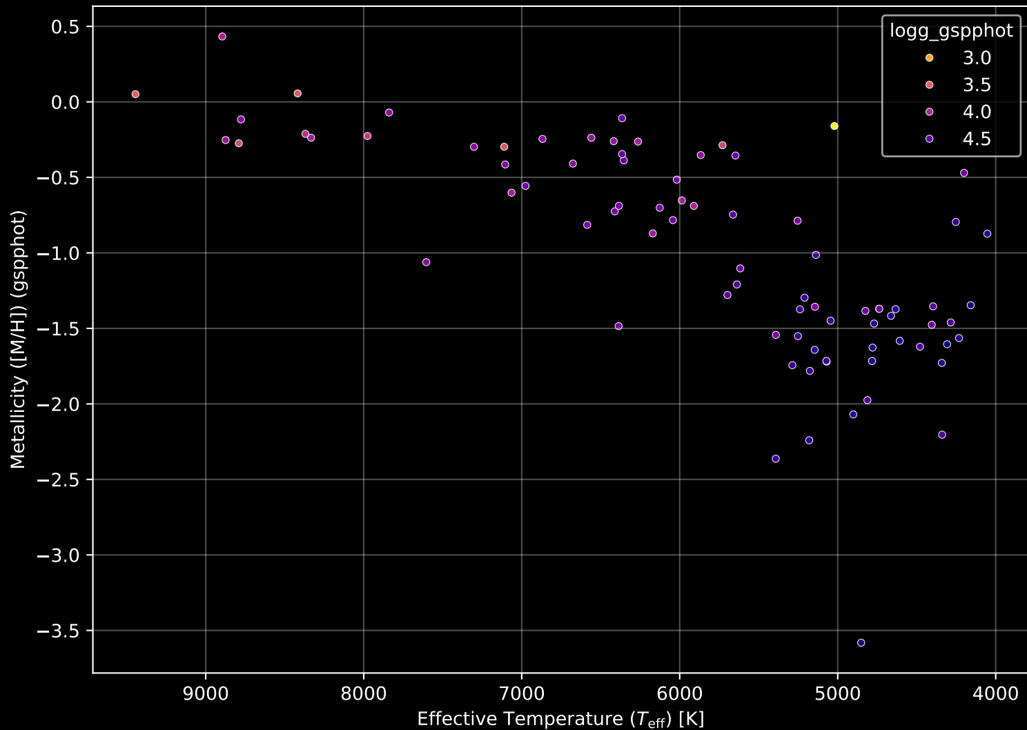
Gaia Cluster: [Gulliver_32] Stellar Population Parameters (n= 81)
