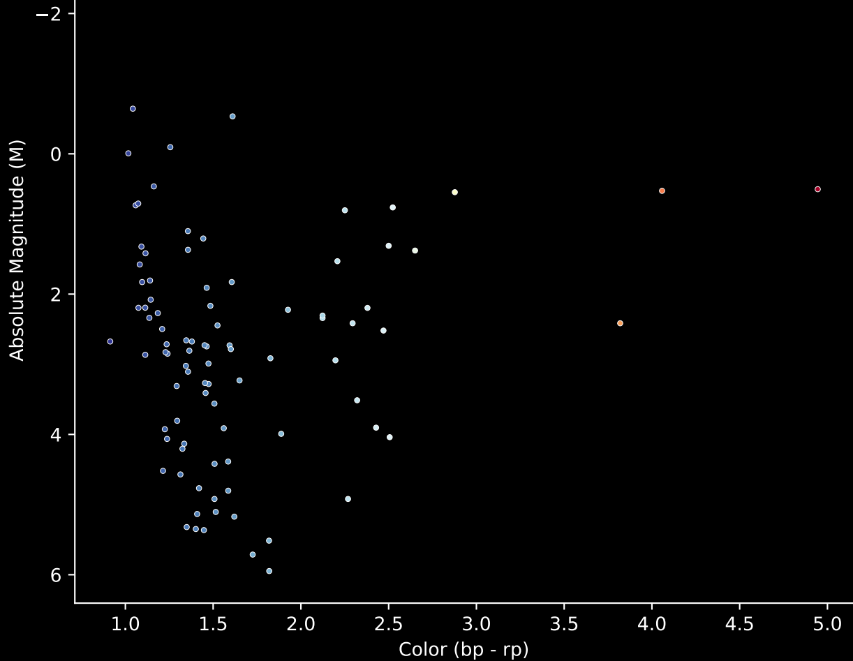
Hertzprung-Russel Diagram
