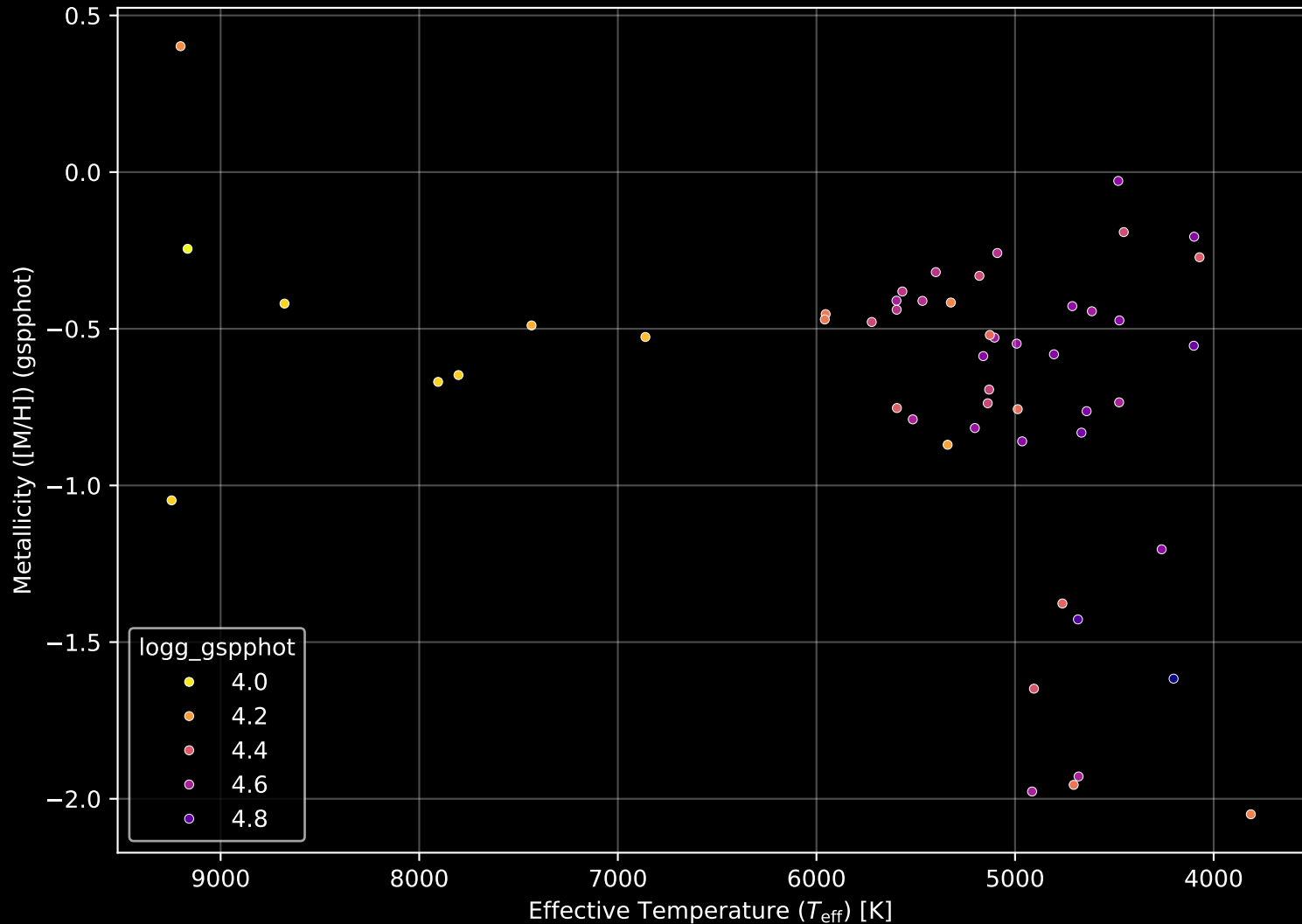
Gaia Cluster: [Gulliver_54] Stellar Population Parameters (n= 52)
