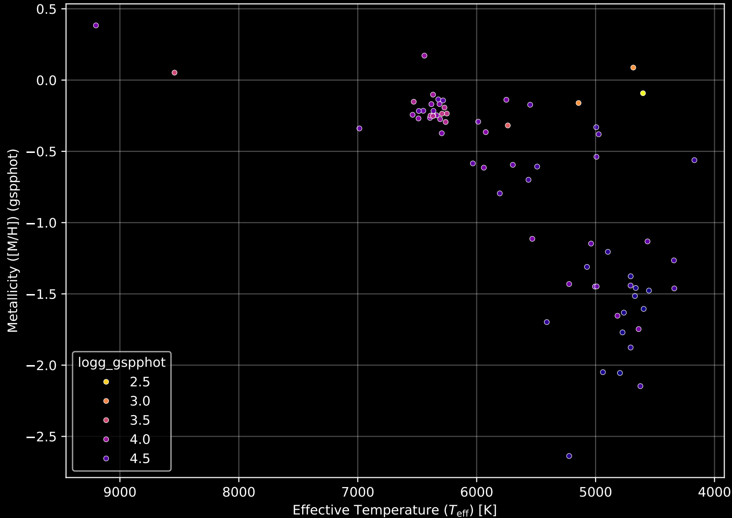
Gaia Cluster: [Gulliver_55] Stellar Population Parameters (n= 70)
