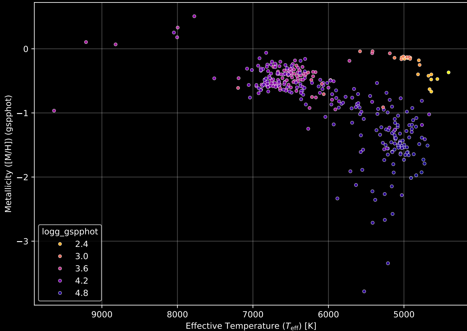
Gaia Cluster: [Haffner_22] Stellar Population Parameters (n= 338)
