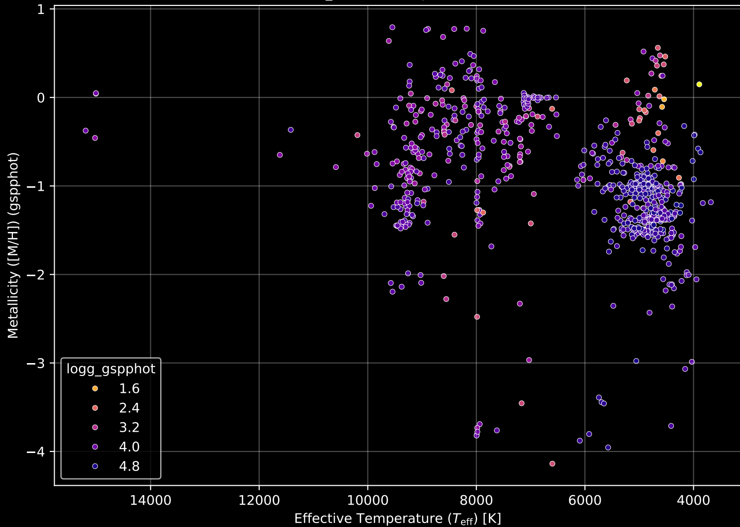
Gaia Cluster: [Harvard_16] Stellar Population Parameters (n= 770)
