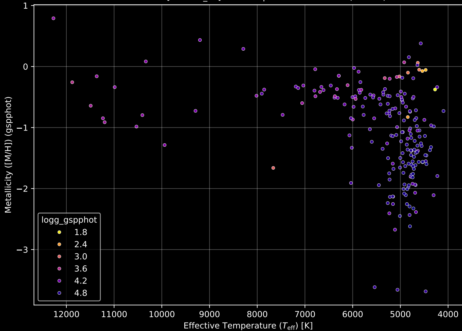
Gaia Cluster: [Harvard_20] Stellar Population Parameters (n= 211)
