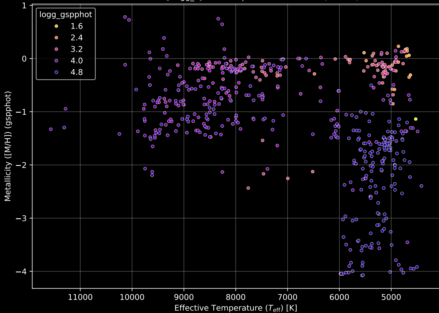
Gaia Cluster: [Hogg_4] Stellar Population Parameters (n= 518)
