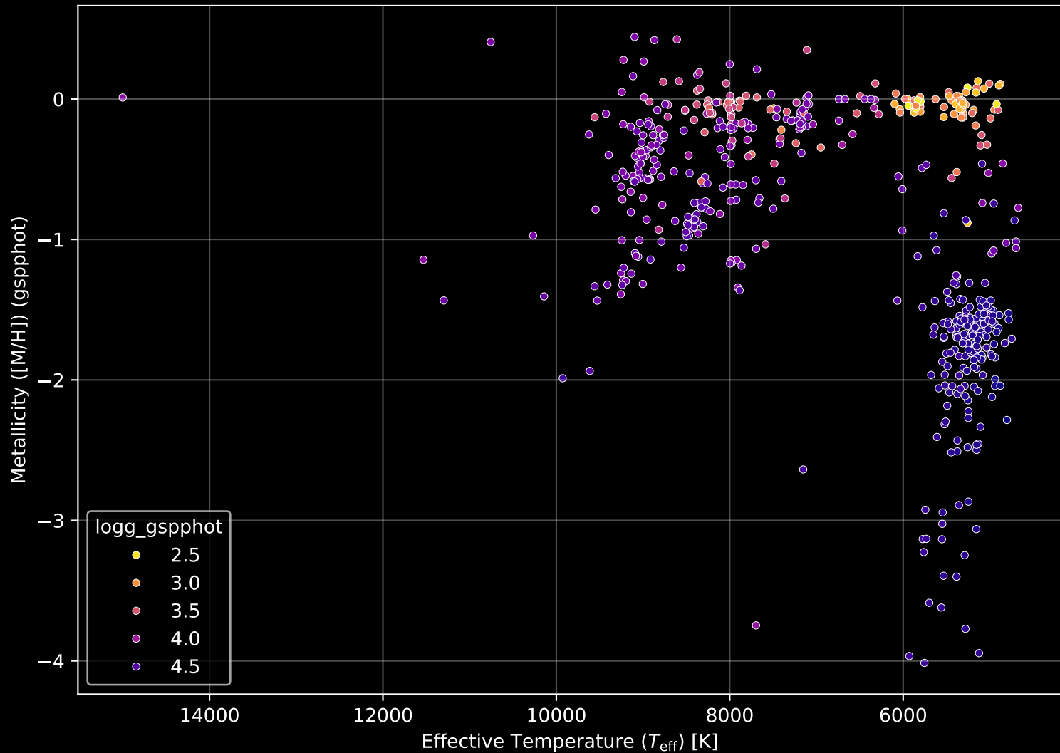
Gaia Cluster: [IC_361] Stellar Population Parameters (n= 545)
