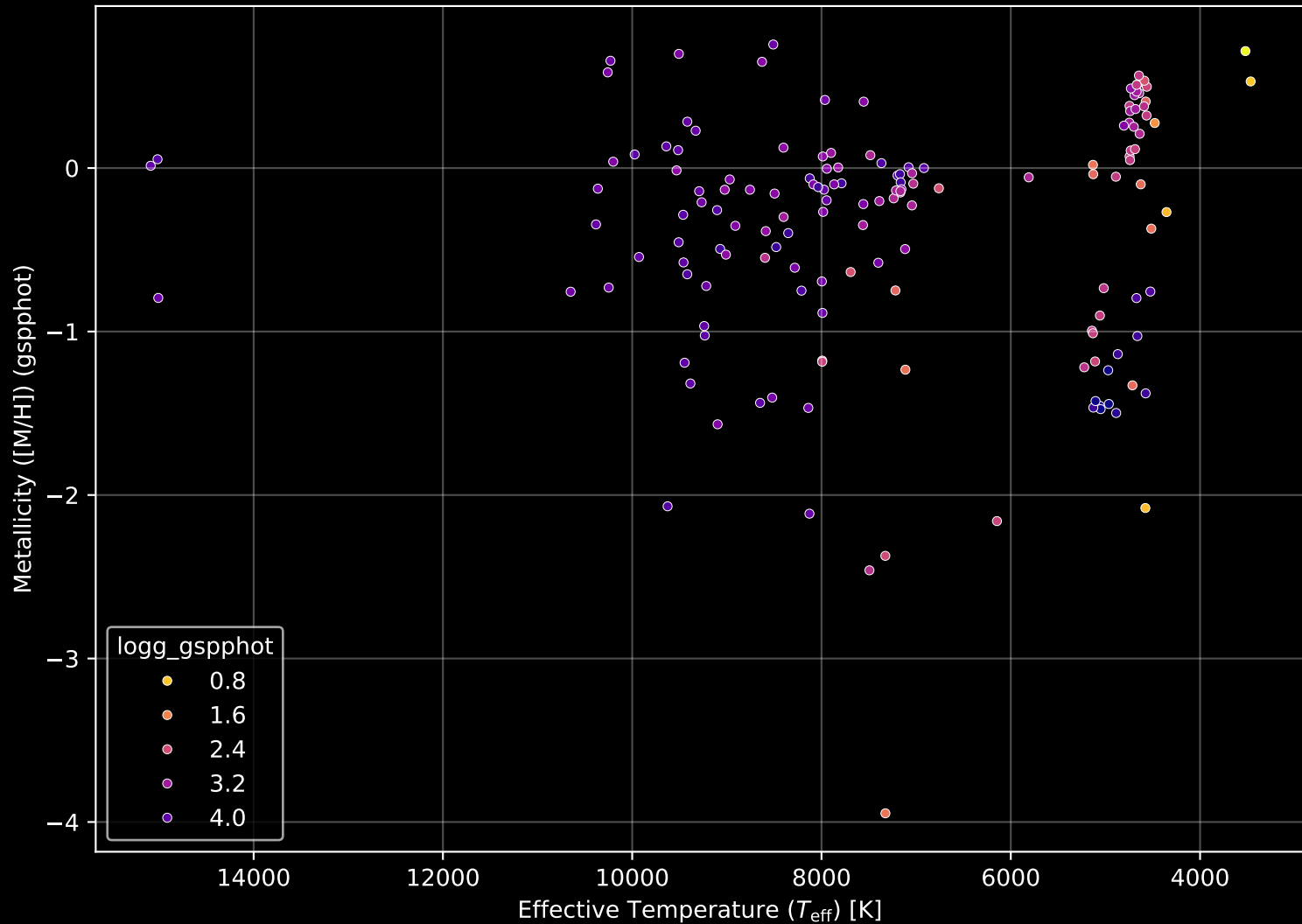
Gaia Cluster: [Juchert_10] Stellar Population Parameters (n= 152)
