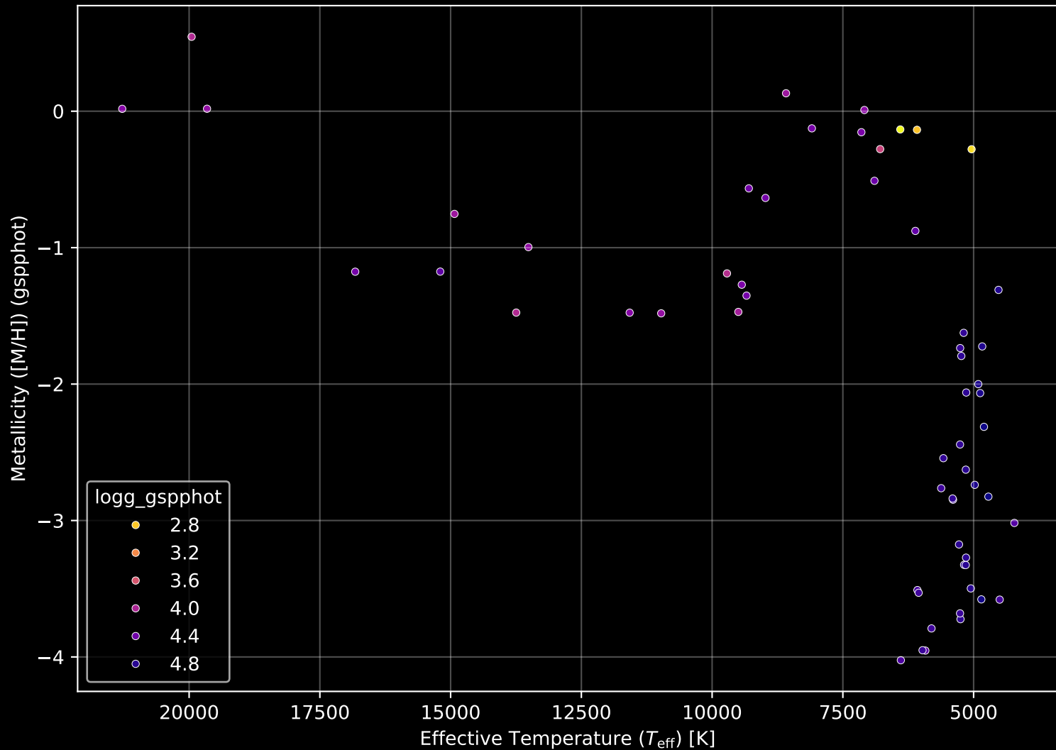
Gaia Cluster: [Juchert_18] Stellar Population Parameters (n= 59)
