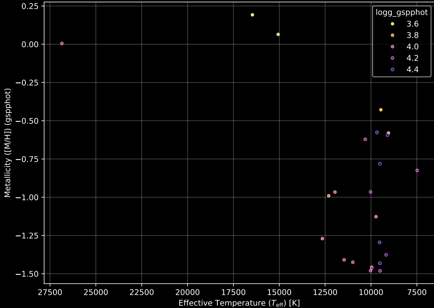
Gaia Cluster: [Juchert_19] Stellar Population Parameters (n= 24)
