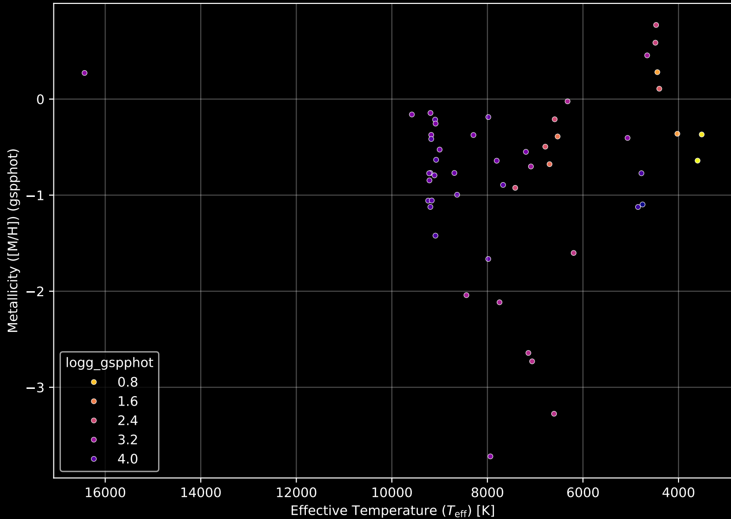
Gaia Cluster: [Juchert_3] Stellar Population Parameters (n= 51)
