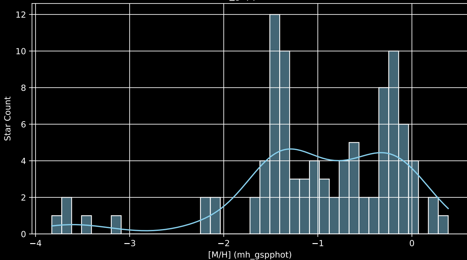
Gaia Cluster: [Juchert_Saloran_1 [M/H] (mh_gspphot) (n= 96)
