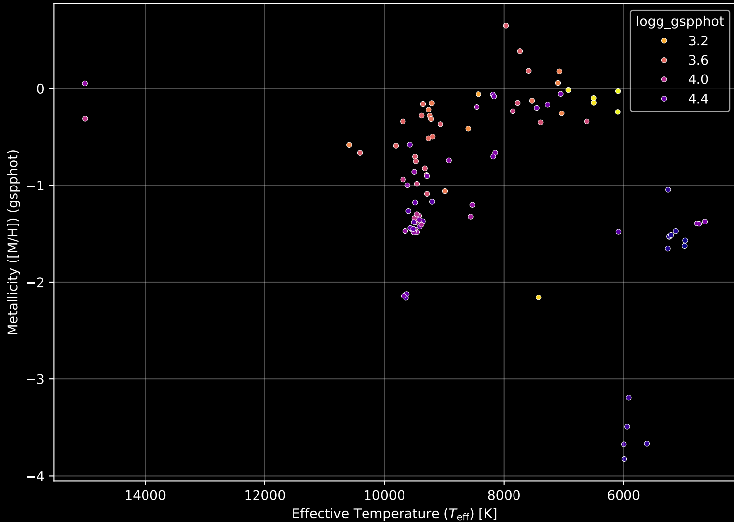
Gaia Cluster: [Juchert_Saloran_1] Stellar Population Parameters (n= 97)
