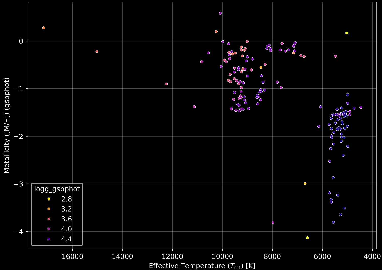
Gaia Cluster: [King_4] Stellar Population Parameters (n= 171)
