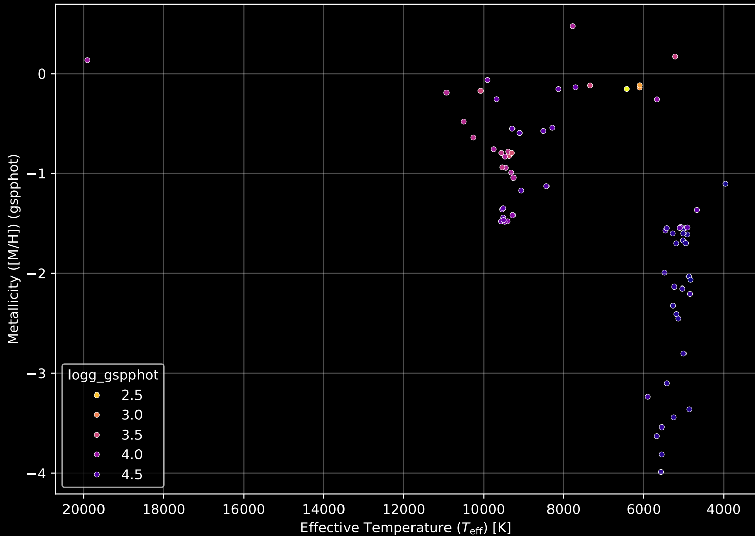
Gaia Cluster: [Koposov_10] Stellar Population Parameters (n= 73)
