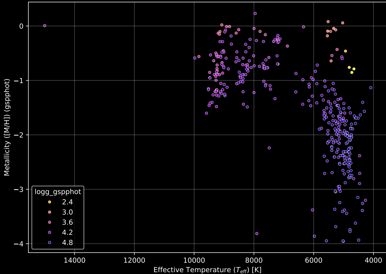
Gaia Cluster: [Koposov_12] Stellar Population Parameters (n= 369)
