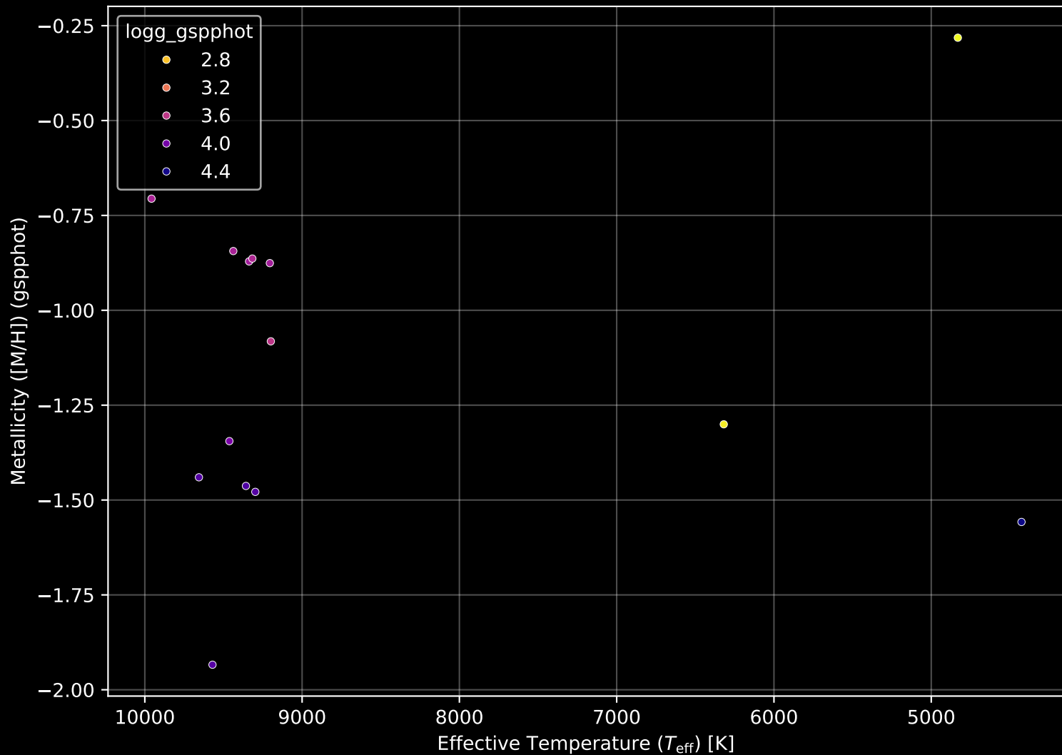
Gaia Cluster: [Kronberger_25] Stellar Population Parameters (n= 14)
